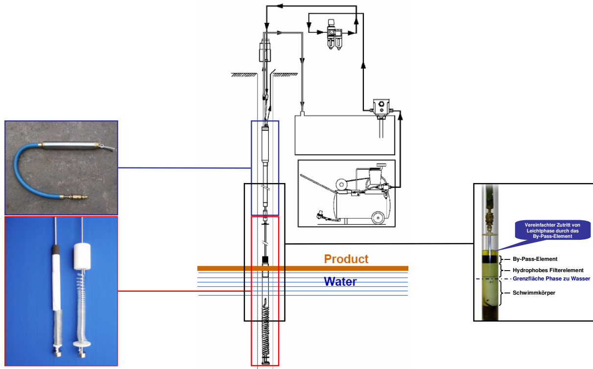
Rückgewinnung von Leichtphase (LNAPL) mit aktivem Skimmersystem
